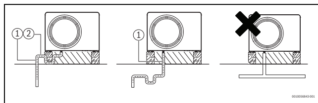
Sl.29 Odvod kondenzata u kanalizaciju / kišni odvod
