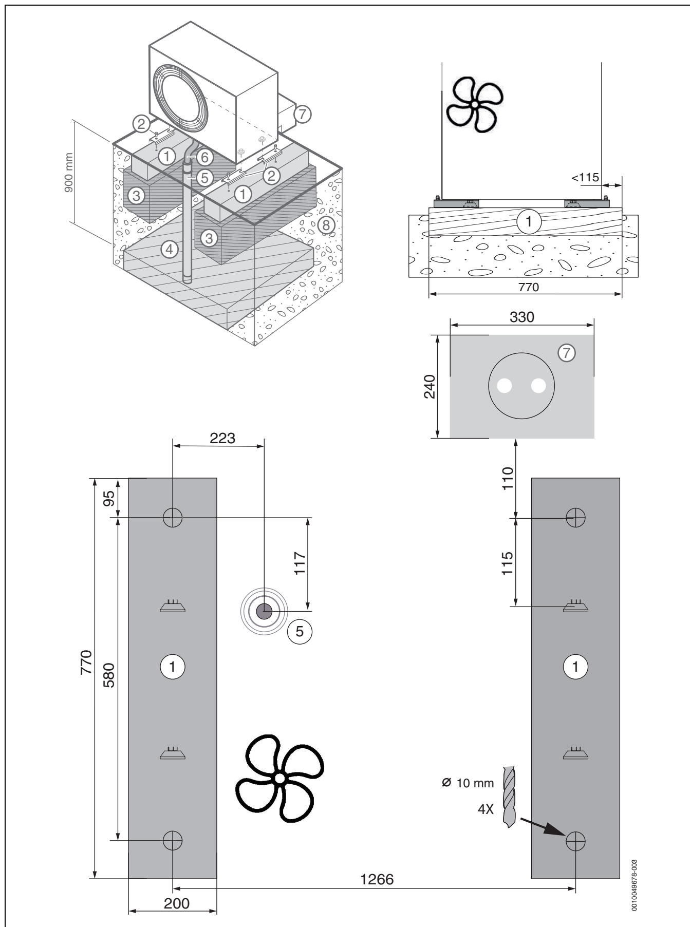
Sl. 24 Plan temelja, alternativa 1
