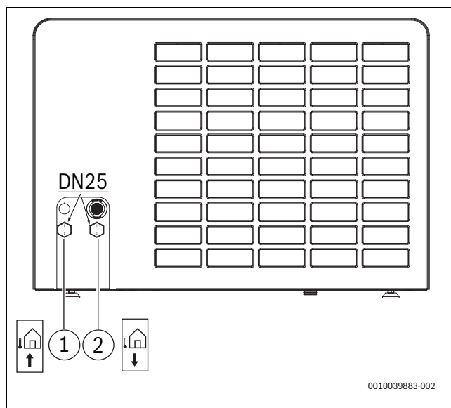
Sl.30 Spojevi cijevi za prijenos topline; opis se primjenjuje na sve veličine
