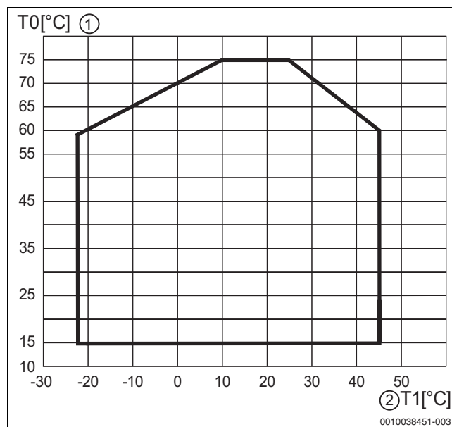
Sl. 44 Dizalica topline u načinu grijanja bez dodatnog grijača
